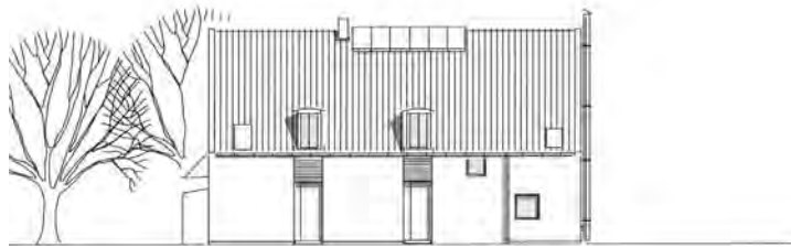
Nordansicht
