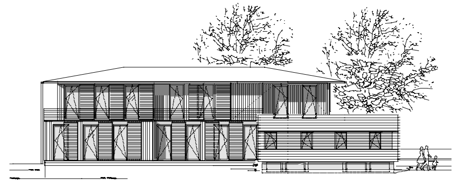
Südansicht
